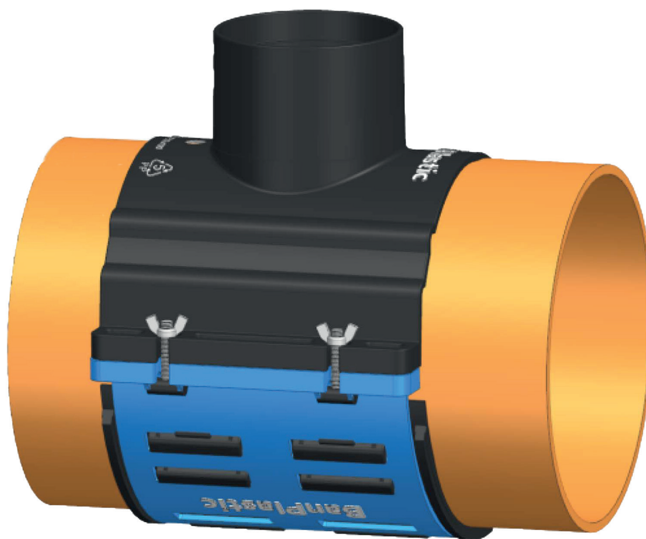
Montagem em tubo de PVC OCRE DN200 mm
